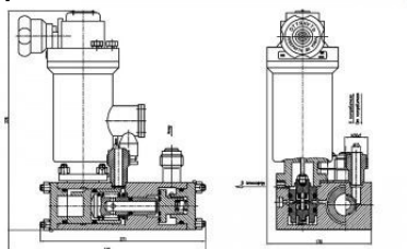
Манипулятор электропневматический 2-х позиционный
